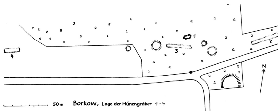
Ryc. 3. Borkowo, gm. Malechowo, stan. 1. Plan cmentarzysk megalitycznego i kurhanowego (Sprockhoff 1964: Taf. 62)
