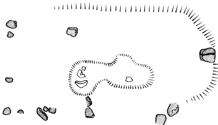
Ryc. 9. Borkowo, gm. Malechowo, stan. 1. Plan grobowca 4 (Sprockhoff 1964: Taf. 62)
