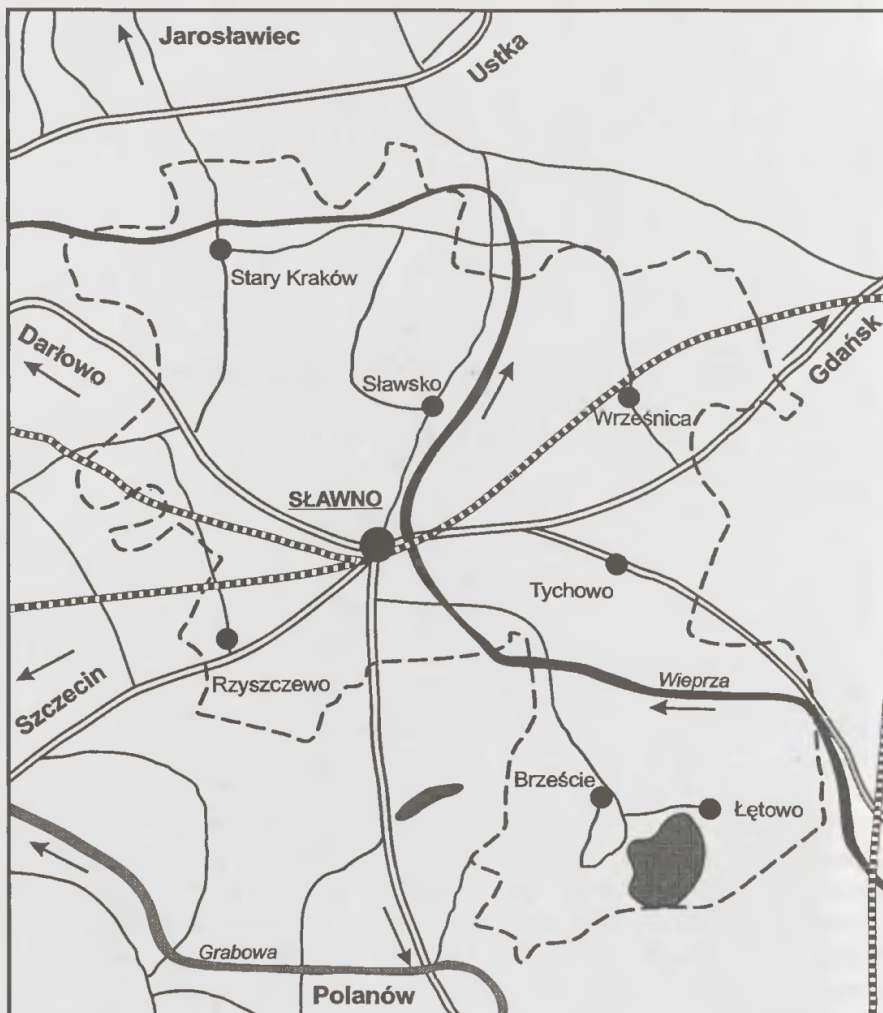
Ryc. 1. Gmina Sławno na tle sieci połączeń komunikacyjnych
